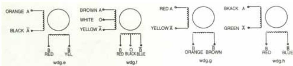
接线图: WIRING DIAGRAM
