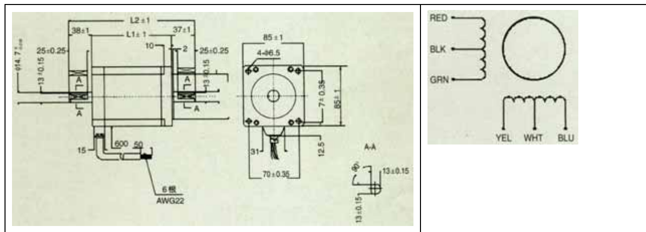
接线图: WIRING DIAGRAM
